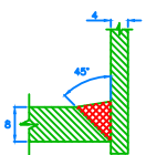
N5 Scale 1:1
